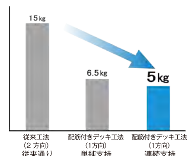
■現場配筋量の比較例(1㎡あたり)
