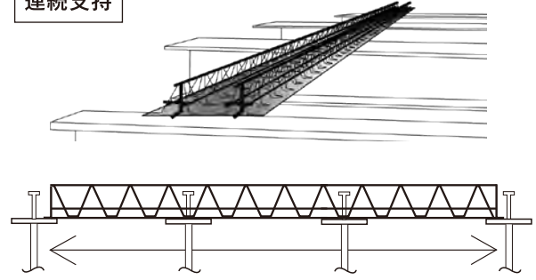
連続支持
