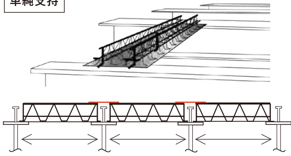
単純支持
